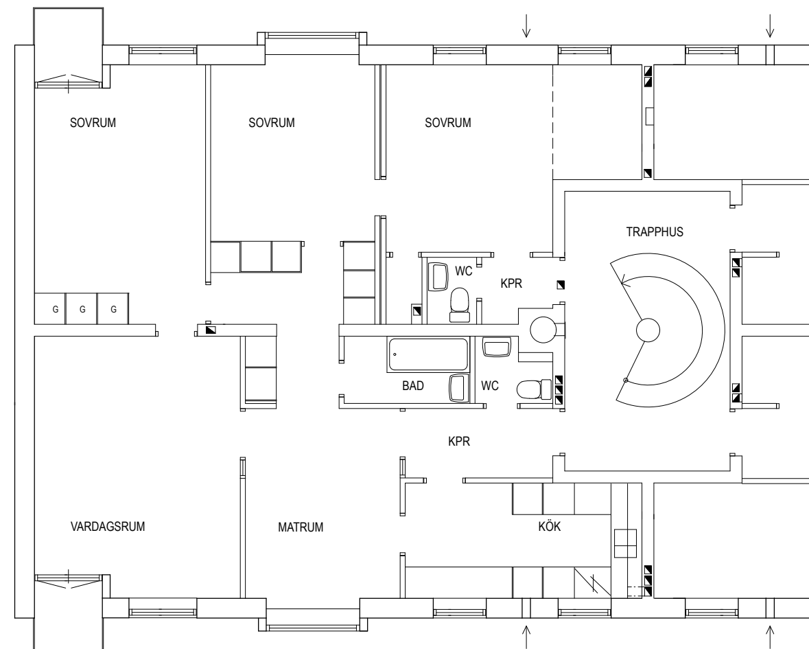
HUS 7 LGH 721-722 PLAN 2
