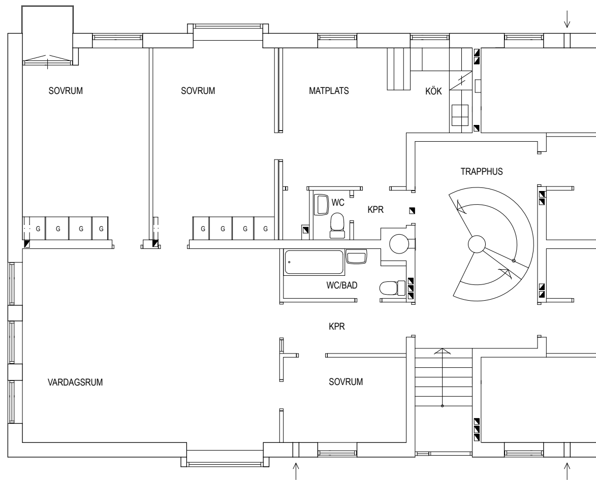
HUS 7 LGH 711-712 PLAN 1
